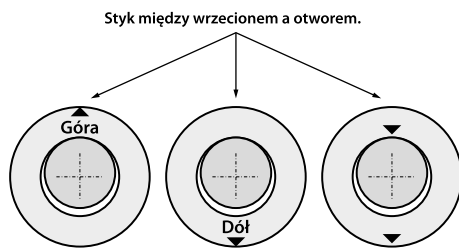
Rys. Przykład znaków określających położenie ściernicy
