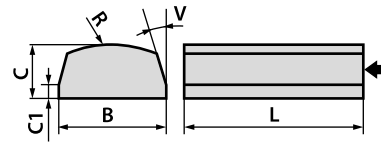
Segment prostokątno - pierścieniowy ścięty 3114 - B \times C / C1 \times L - R...V...
