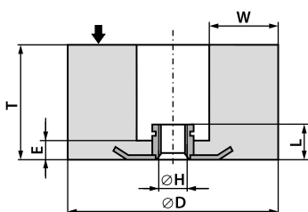
Ściernica garnkowa walcowa z wkładką gwintową 6002 - D × T × H / L - W...E...
