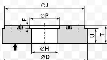
Ściernica tarczowa z wkładkami gwintowymi i wybraniem walcowym od strony mocującej 3603 - D × T × H - nr rysunku
