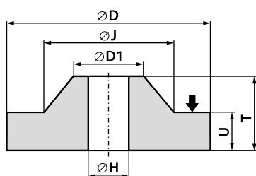
3802 - D / J x T / U x H - nr rysunku
