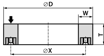
37 - D x T - W... - nr rysunku W < 0,17D
