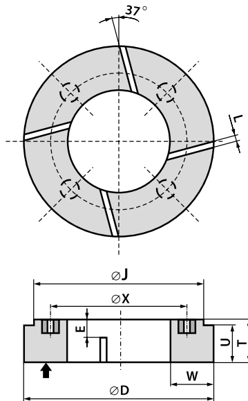
3701 - D x T - W... - nr rysunku W < 0,17D
