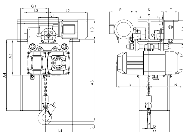
Model YaleVego CPV/CPVF stałe połączenie z wózkiem elektrycznym
