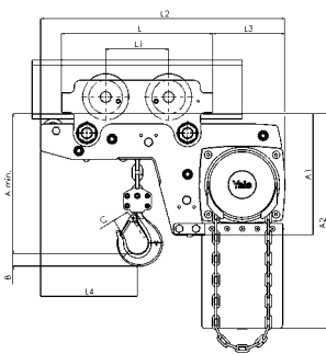
Model Yalelift LHP, 500 - 3.000 kg, z jednym ciągnem
