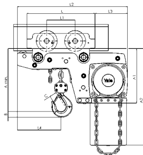
Model Yalelift LHG, 500 - 3.000 kg, z jednym ciągnem
