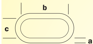
Wymiary ogniwa pokrytego
