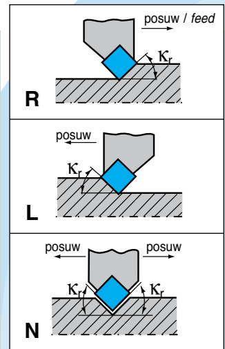
Kierunek skrawania 5 Cutting direction
