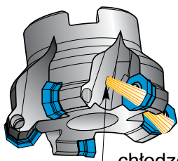
chłodzenie coolant
